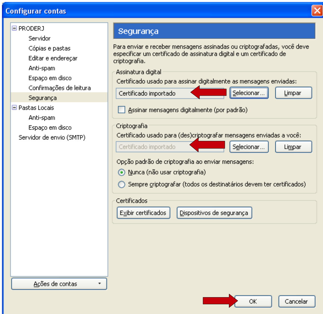
Figura 20: Certificado já vinculado à conta de email do usuário. Clique em OK.
